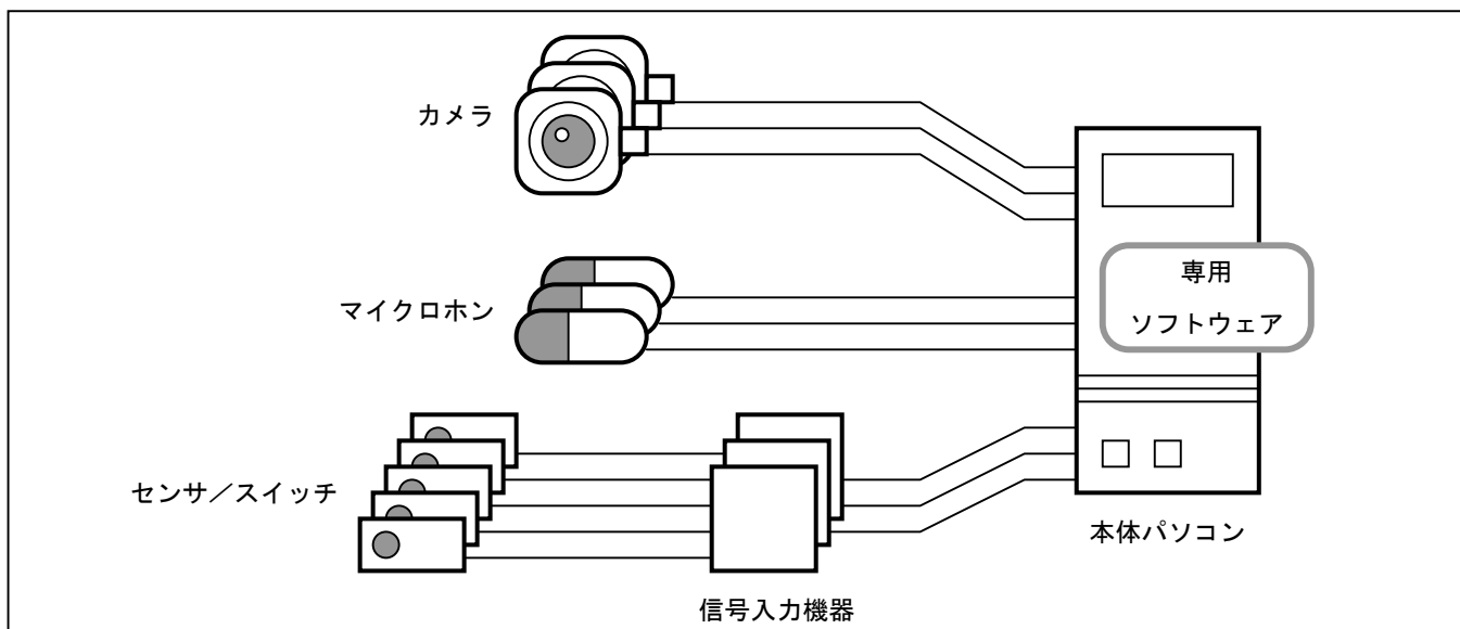
図. 「コスモレコーダー」のシステム構成
